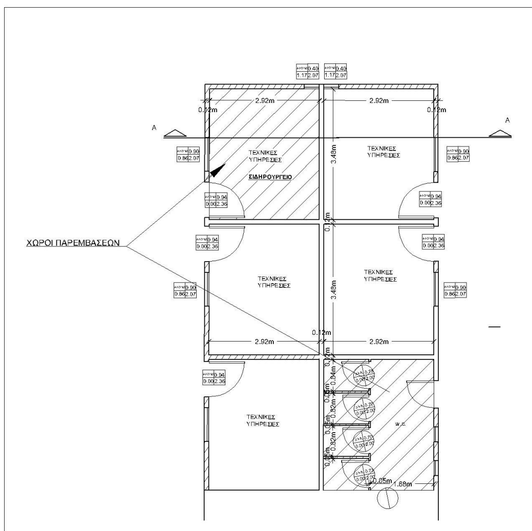
Σχέδιο 1 : Κάτοψη χώρου Παρεμβάσεων.
